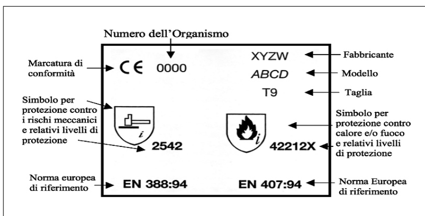
Esempio di marcatura di un quanto di protezione per rischi meccanici e da calore e/o fuoco
