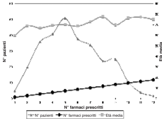
Figura 1. Correlazioni pluriprescrizione/età.
